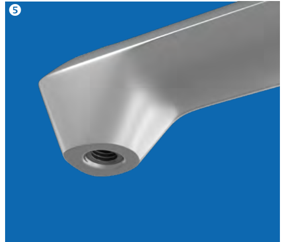
5 Nach Abkühlung der erstarrten Schmelze erhalten Sie ein verschleißfreies, belastbares Gewinde in Ihren hochwertigen Leichtmetallbauteilen.
