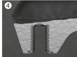
4 Die flüssige Aluminiumschmelze füllt die Form aus und umschließt den HELICOIL® Cast, ohne in das Innengewinde einzuströmen.
