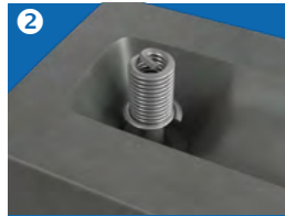
2 Aufstecken des HELICOIL® Cast auf den glatten Kernstift
