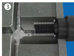
3 Die unter hohem Druck eingepresste flüssige Aluminiumschmelze füllt die Form aus und umschließt den HELICOIL® Cast auf dem Spindelkern, ohne in das Innengewinde einzuströmen.
