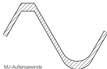
MJ-Außengewinde
