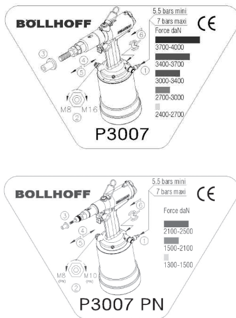
Figura 8 - Regolazione
