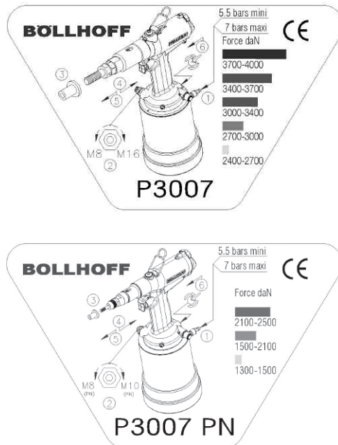
Abbildung 8 - Einstellhilfe
