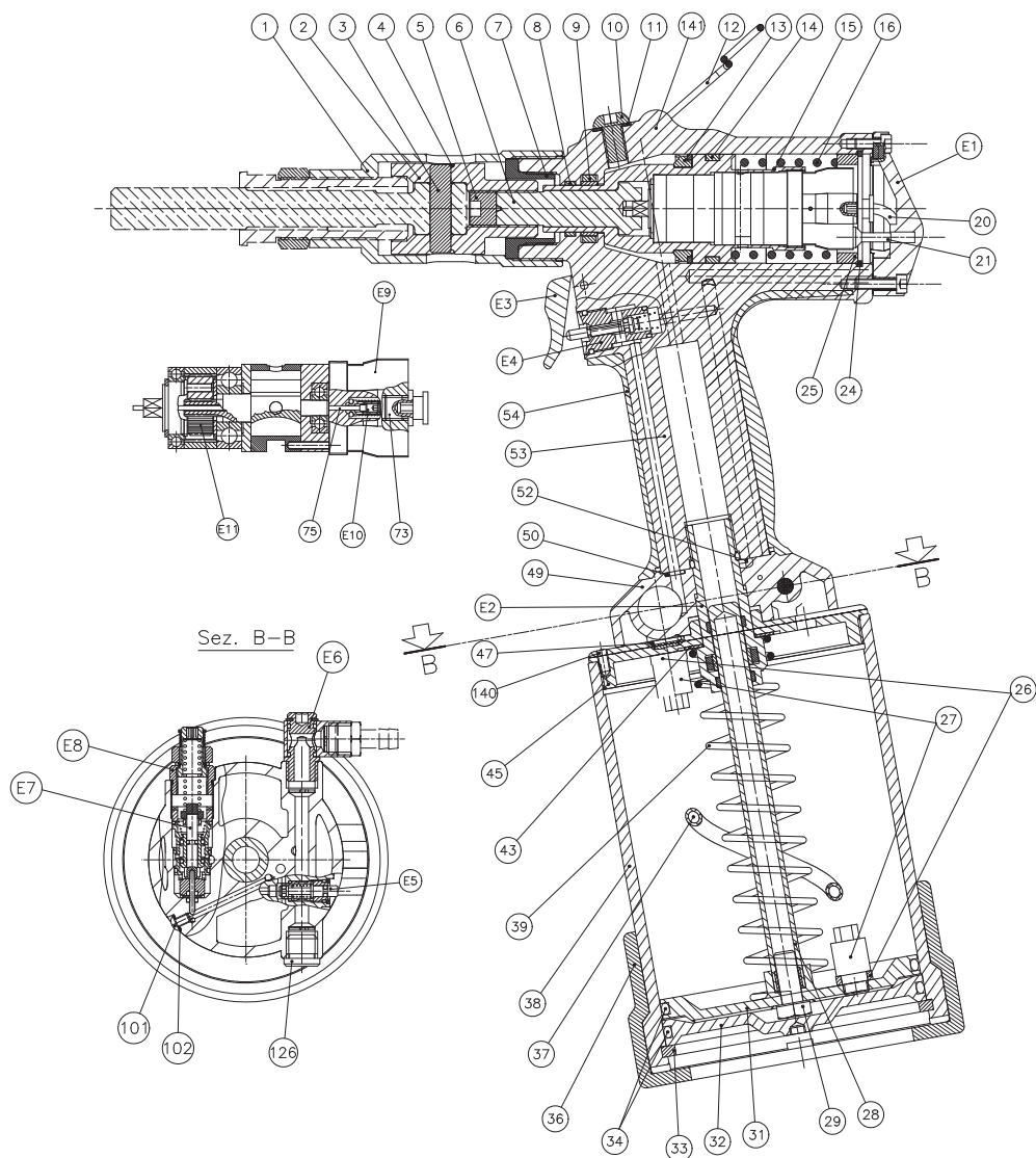
Figura 11 - Despiece
