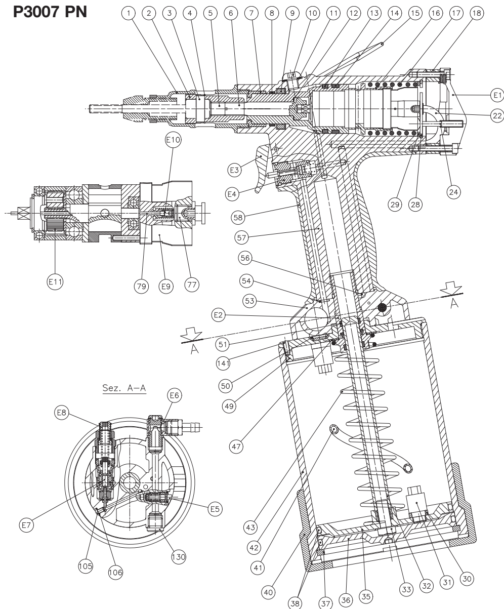
Abbildung 12 - Ersatzteileübersicht
