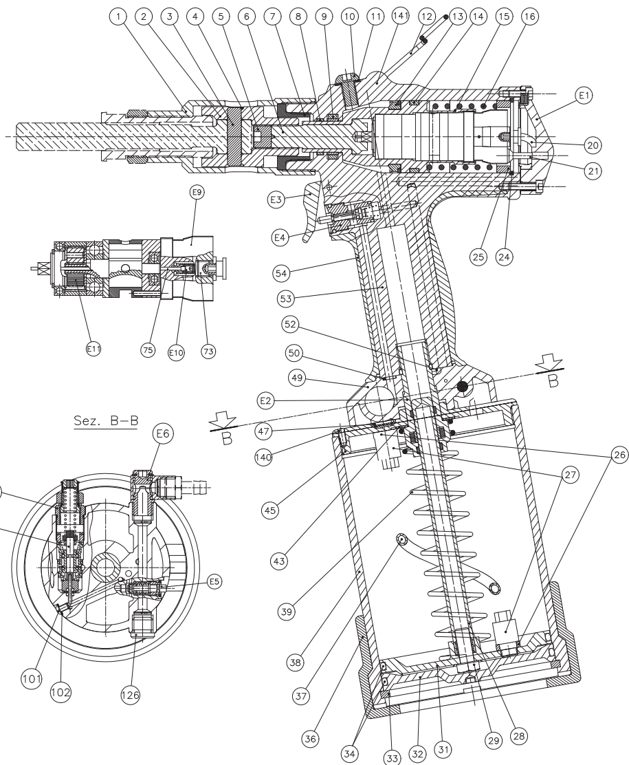
Abbildung 11 - Ersatzteileübersicht
