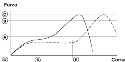
Figura 3 - Grafico forza/corsa
