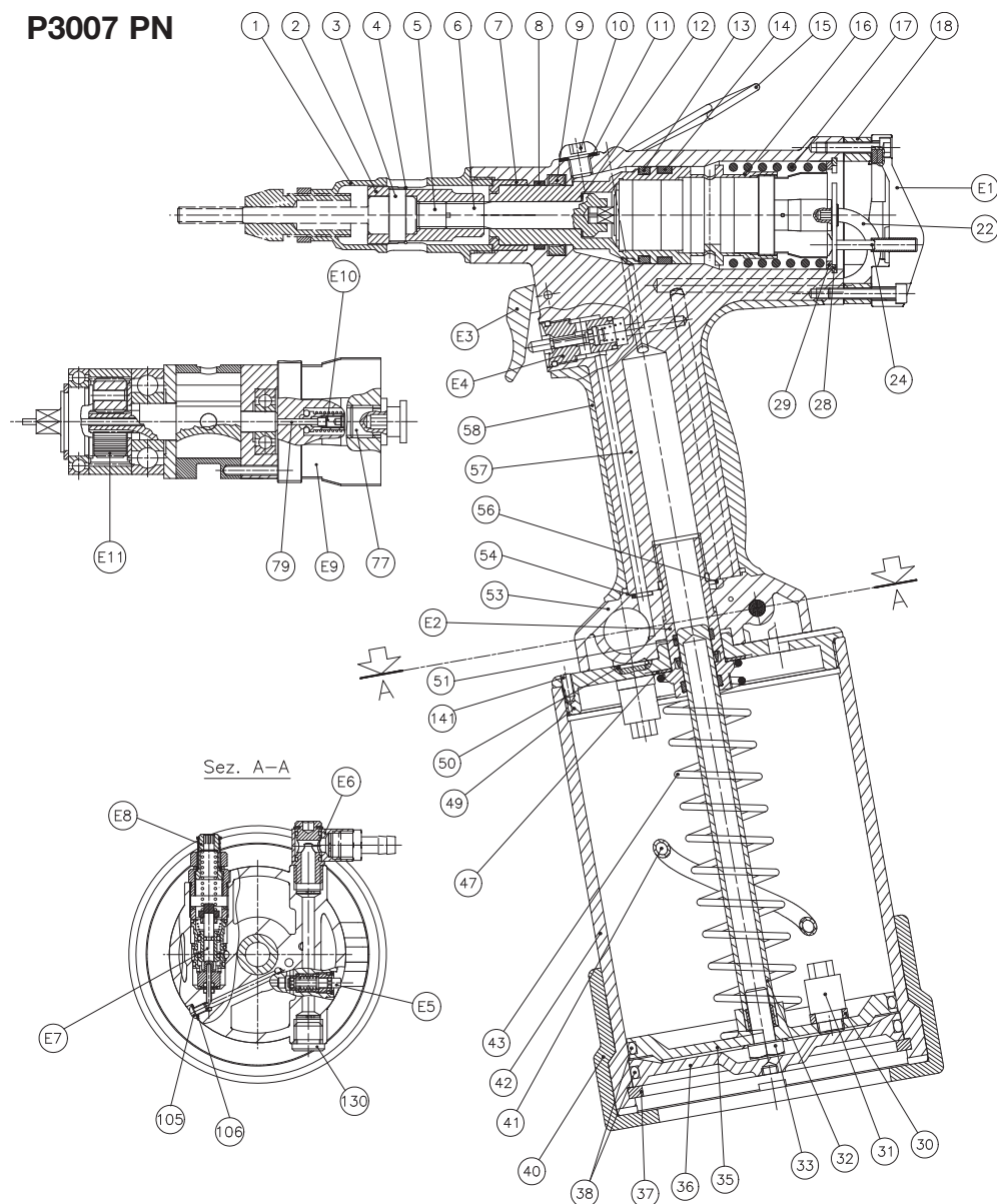
Figura 12 - Despiece
