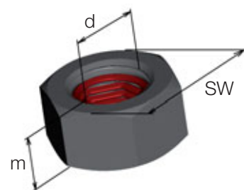
Sechskantmutter, ähnlich DIN 934
