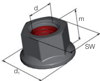
Bundmutter, ähnlich DIN 6923
