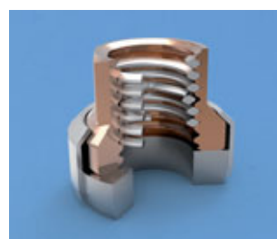
HELICOIL® Sicherungsmutter als Bundmuttervariante mit Scheibe
