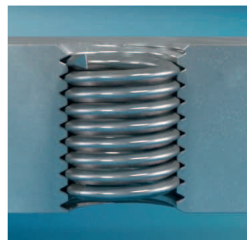
Installation correcte de l'HELICOIL® Tangfree entre 0,25 et 0,50 pas en-dessous de la surface de la pièce
