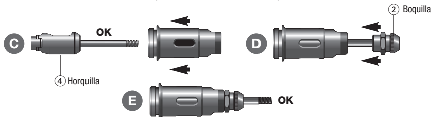
Figura 4 - Alineación del vástago
