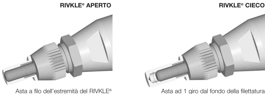
Figura 5 - Regolazione della posizione del nasello con controdamo
