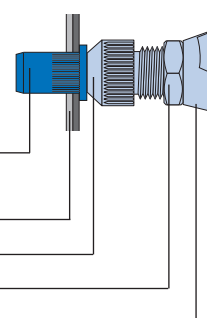
RIVKLE® blind rivet stud
