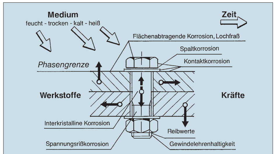
Prinzipielle Darstellung des „Korrosionssystems Schraubverbindung“ mit seinen wesentlichen Funktionsgrößen und Beispielen von möglichen Korrosionsarten
